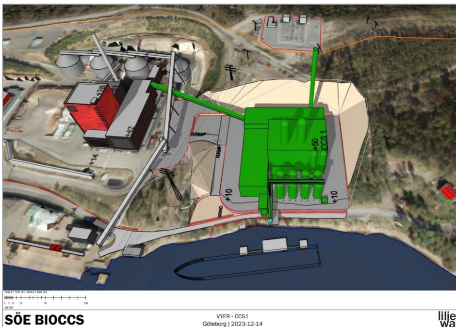
Figur 2 Planerad CCS-anläggning (i grönt) och Igelsta kraftvärmeverk
